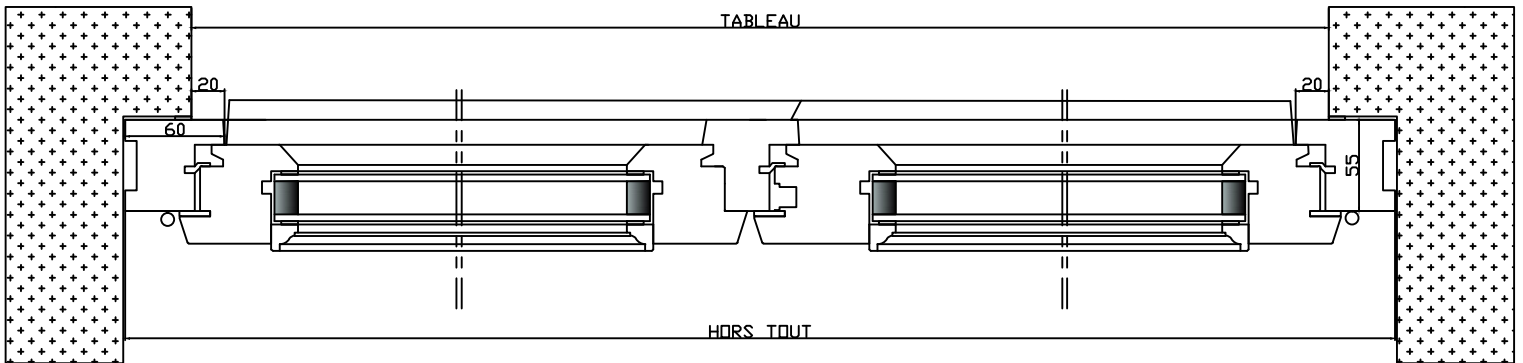
Porte fenêtre à 2 vantaux à recouvrement
